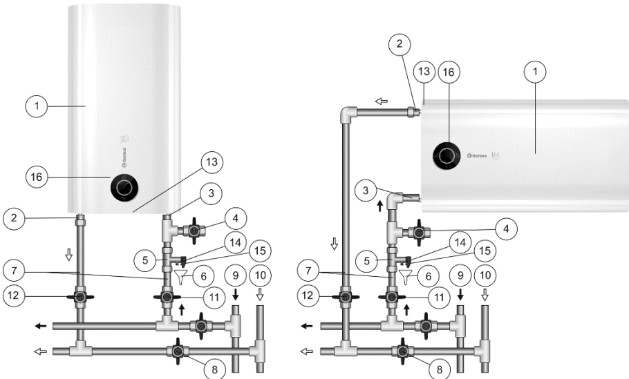
Bild 1. Wasseranschluss
