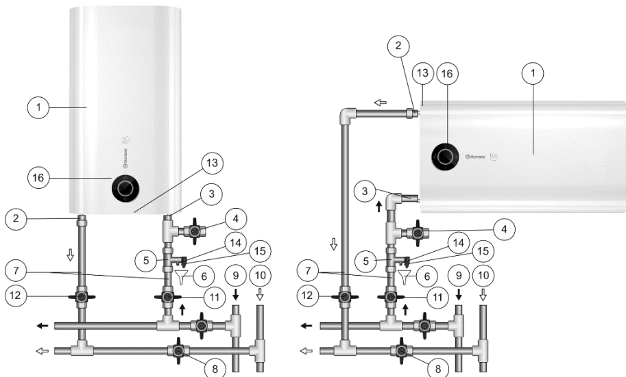
Рисунок 1. Схема подключения ЭВН к водопроводу
