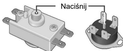
Ilustr. 3. Plan rozmieszczenia przycisku wyłącznika termicznego
