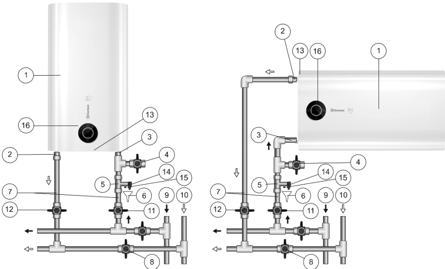
Attēls 1. EŪS pieslēgšana pie ūdensapgādes tīkla
