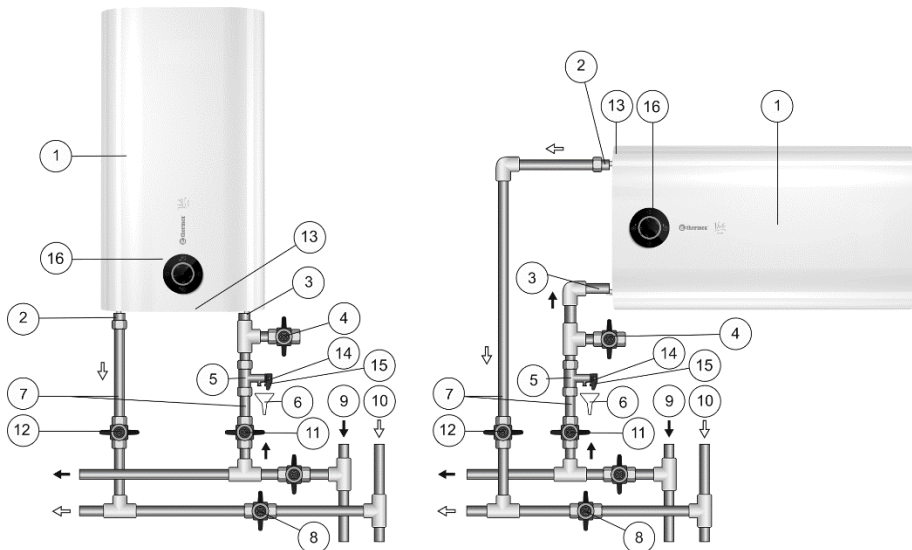
Paveikslas 1. EVŠ prijungimo prie vandentiekio schema
