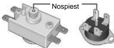
Attēls 3. Termoslēdzēja pogas novietošanas
