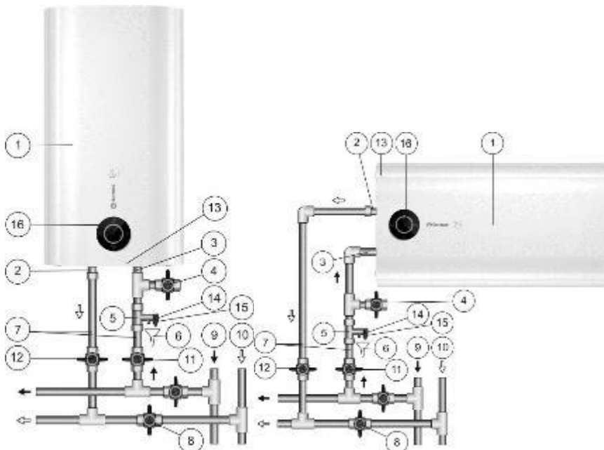
Ilustr. 1. Przyłącze wodne
