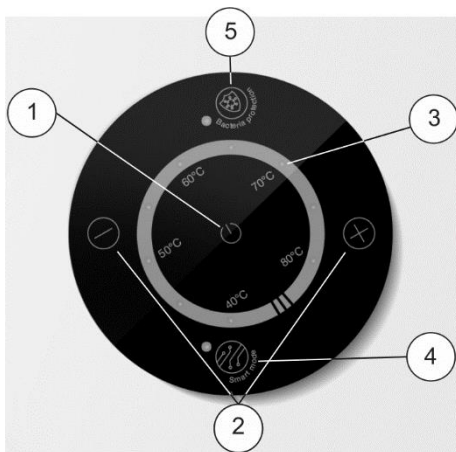
Paveikslas 2. Elektrinė valdymo panelė
