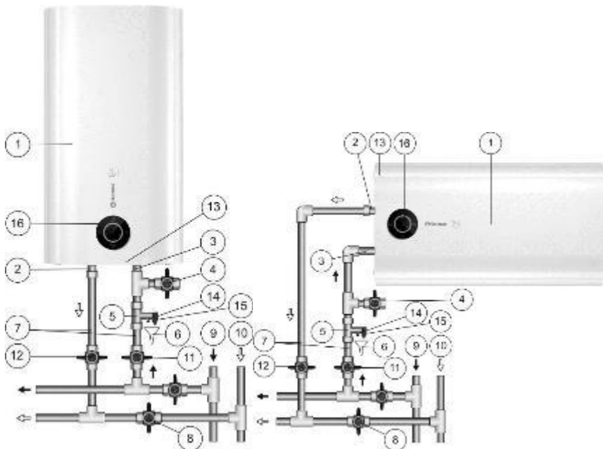
Kuva 1. Kaavio SVL:n liittämistä vesiverkkoon
