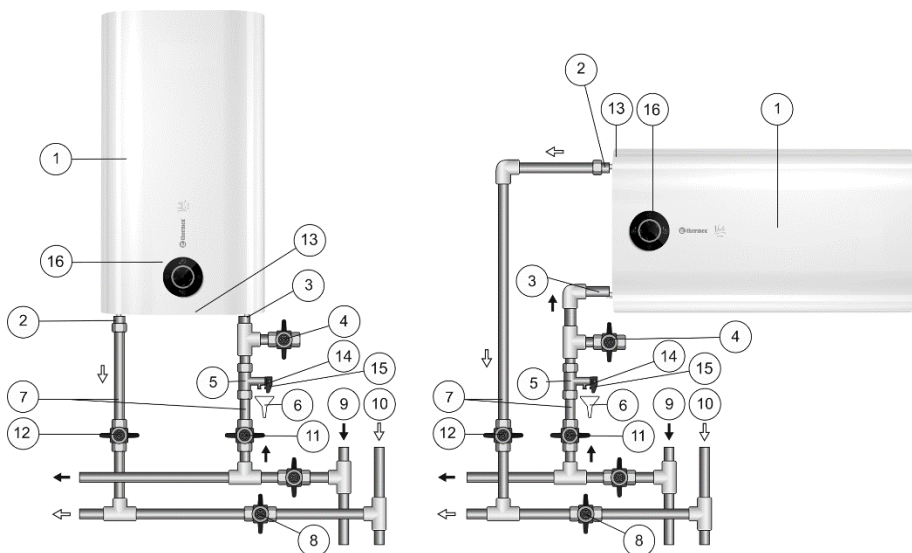
Joonis 1. Veeboileri veevõrguga ühendamise skeem
